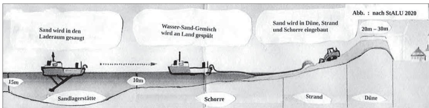
Schematische Darstellung einer Sandaufspülung von See aus
